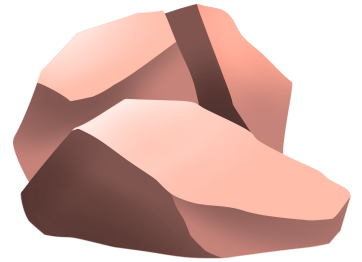
roter Buntsandstein
