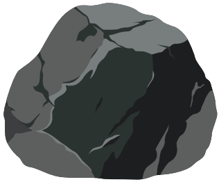
schwarzer Basalt
